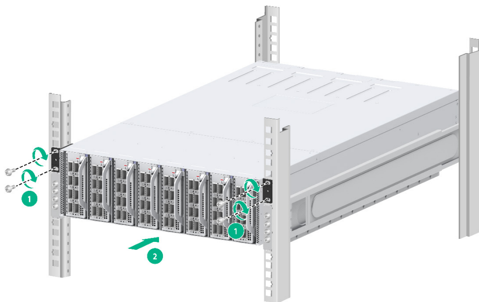
图2-10 安装 S9800XP-8C-G 交换机到机柜示意图
