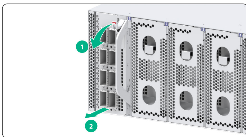
图2-28 接口模块扩展卡拆卸示意图
