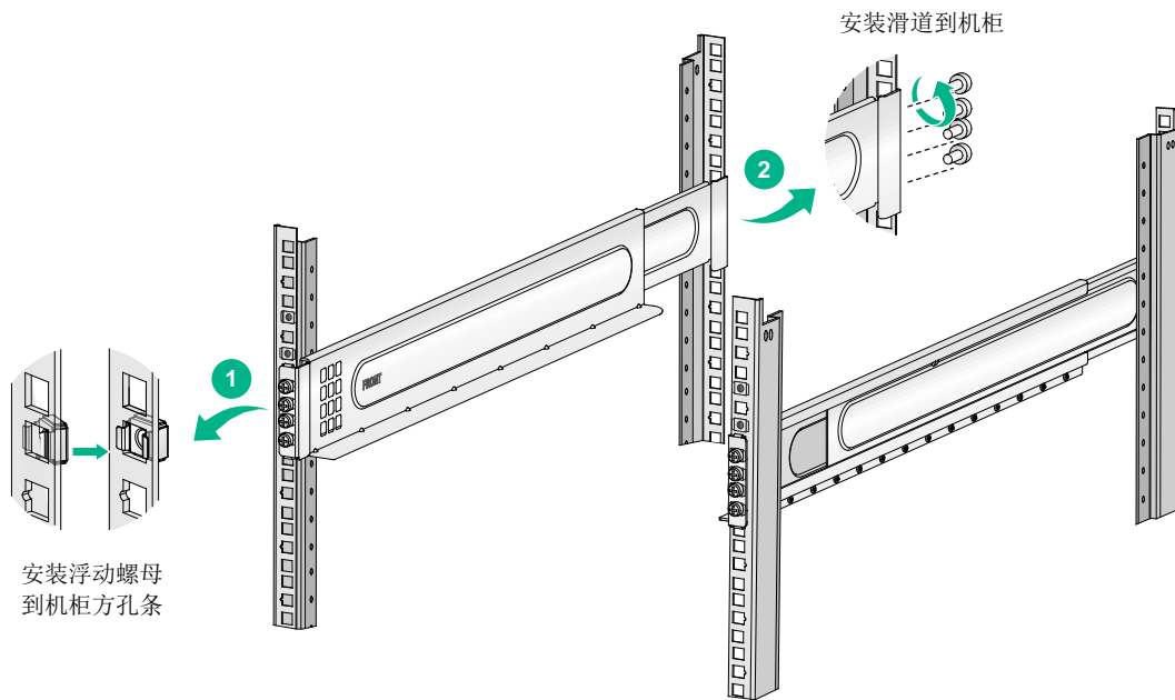
图2-9 S9800XP-8C-G 浮动螺母与滑道安装示意图
