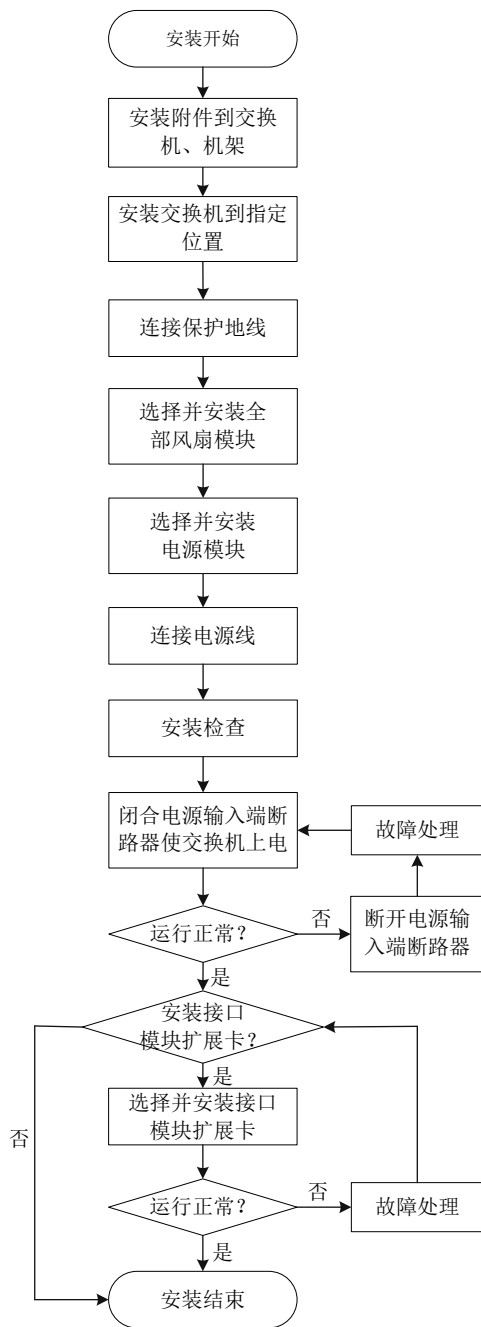
图2-1 交换机安装流程
