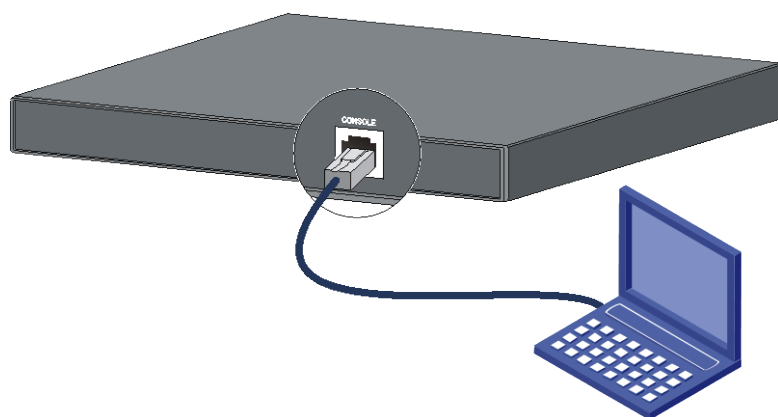
图3-1 交换机初次上电启动配置组网图（串行配置口电缆连接）
