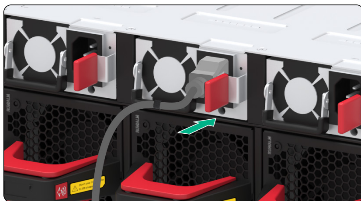
图2-24 PSR2000-12A-S-Z 交流电源线连接示意图
