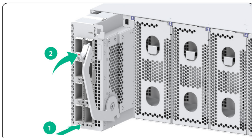
图2-27 接口模块扩展卡安装示意图
