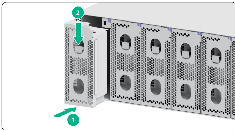
图2-29 接口模块扩展卡假面板安装示意图
