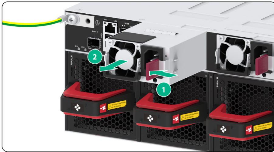
图2-22 拆卸电源模块示意图
