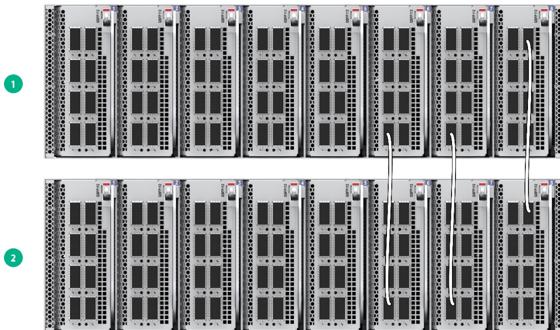
图4-2 M-LAG 连接示意图
