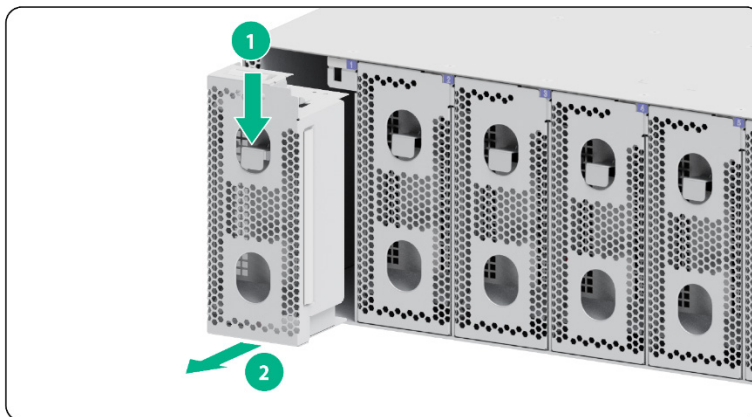
图2-25 接口模块扩展卡假面板拆卸示意图
