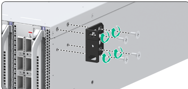
图2-8 安装挂耳到 S9800XP-8C-G 机箱的示意图
