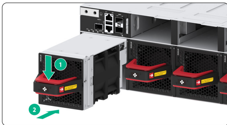
图2-15 风扇模块安装示意图
