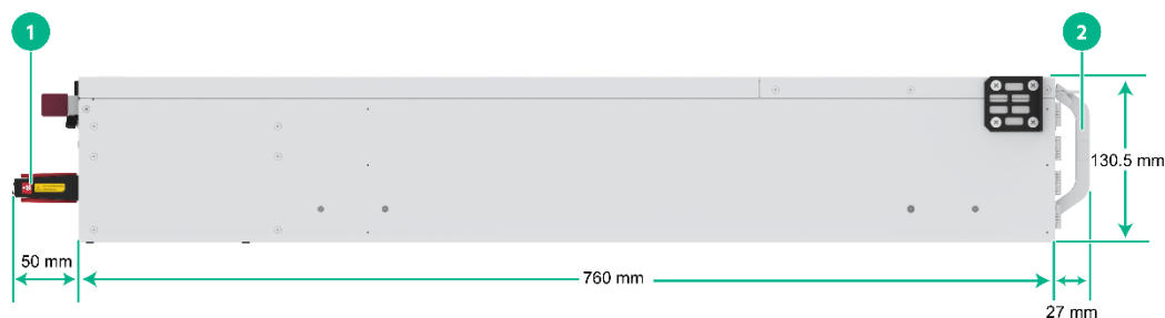
图2-3 S9800XP-8C-G 交换机尺寸示意
