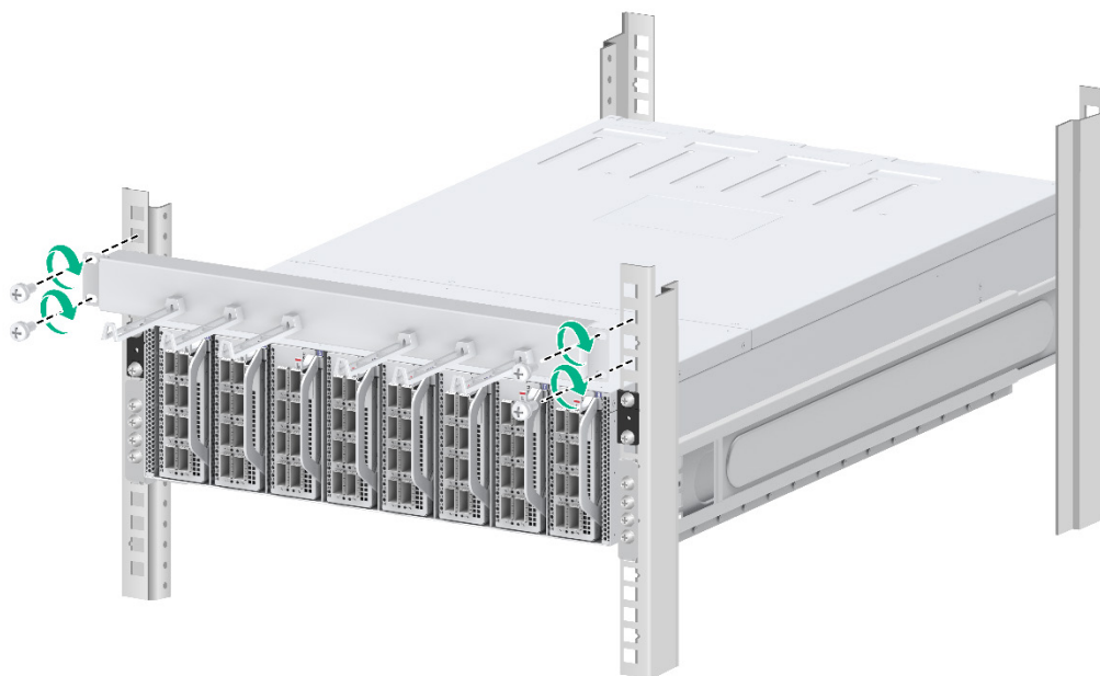
图2-11 安装走线架到机柜示意图
