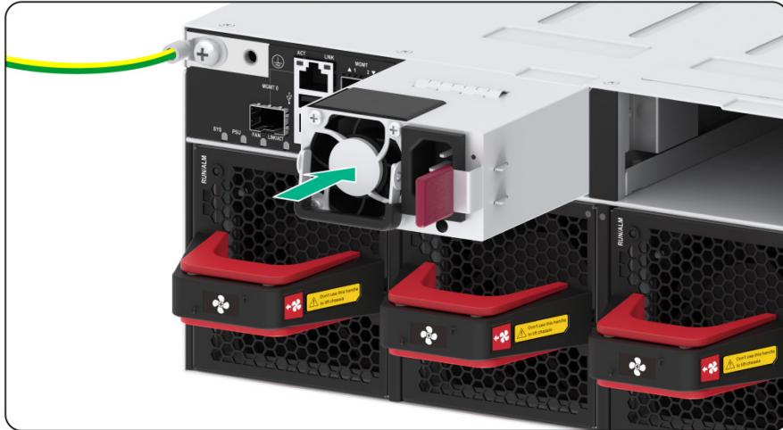
图2-20 电源模块安装示意图
